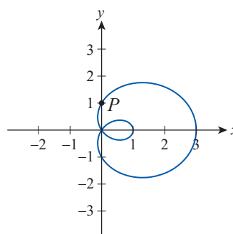
Limaçon
