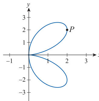
Bifolium
